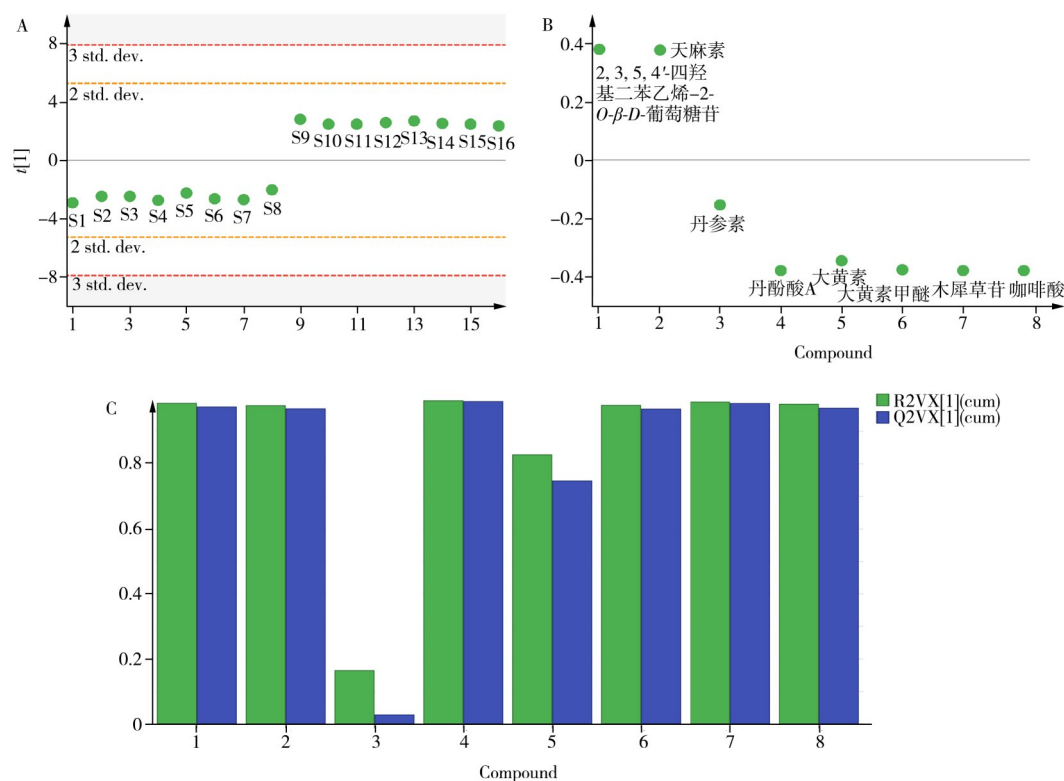
图 4 16 批样本的 PCA 分布散点图(A)、载荷图(B)与各成分贡献率(C)
