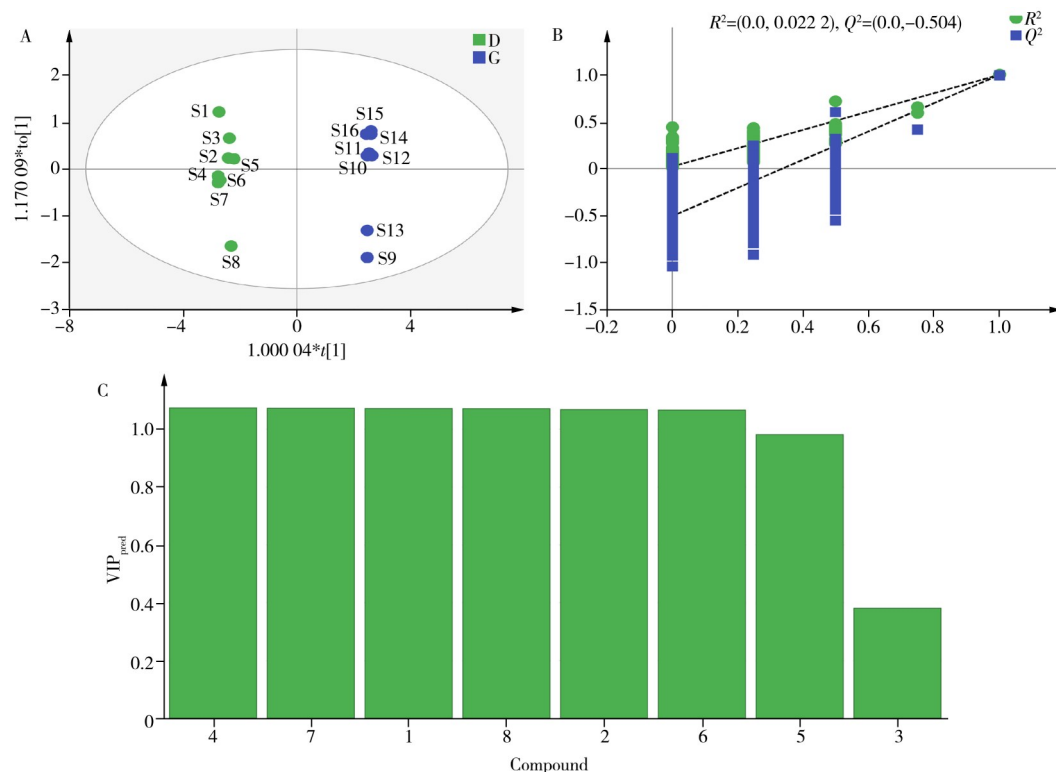
图 5 16 批样本的 OPLS-DA 分布散点得分图(A)、置换检验图(B)与 VIP 值(C)
