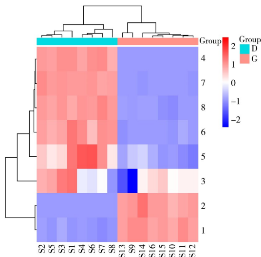
图3 16 批 TMSC 样品中 8 种成分的聚类分析 Fig. 3 Cluster analysis of 8 components in 16 samples of TMSC
